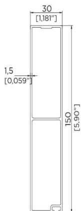
30X150 BOX PROFILE
